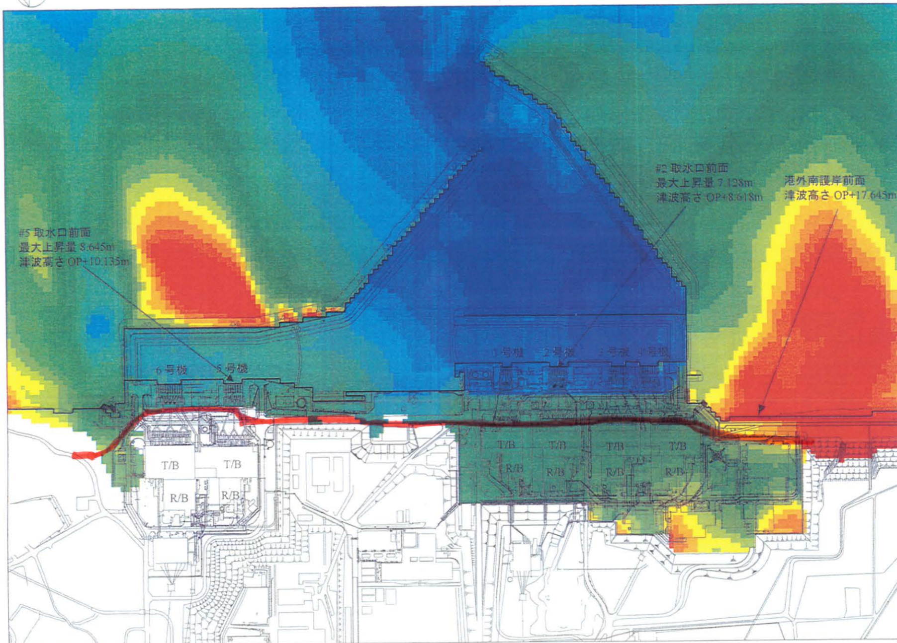
図 2-4 1F 詳細パラスタ 最大津波高さ分布 上昇側最大値ケース (R9-06-02H, 朔望平均満潮位時 OP+1.490m)
