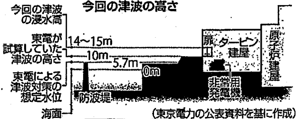
◆福島第一原発で想定された津波の高さと今回の津波の高さ
