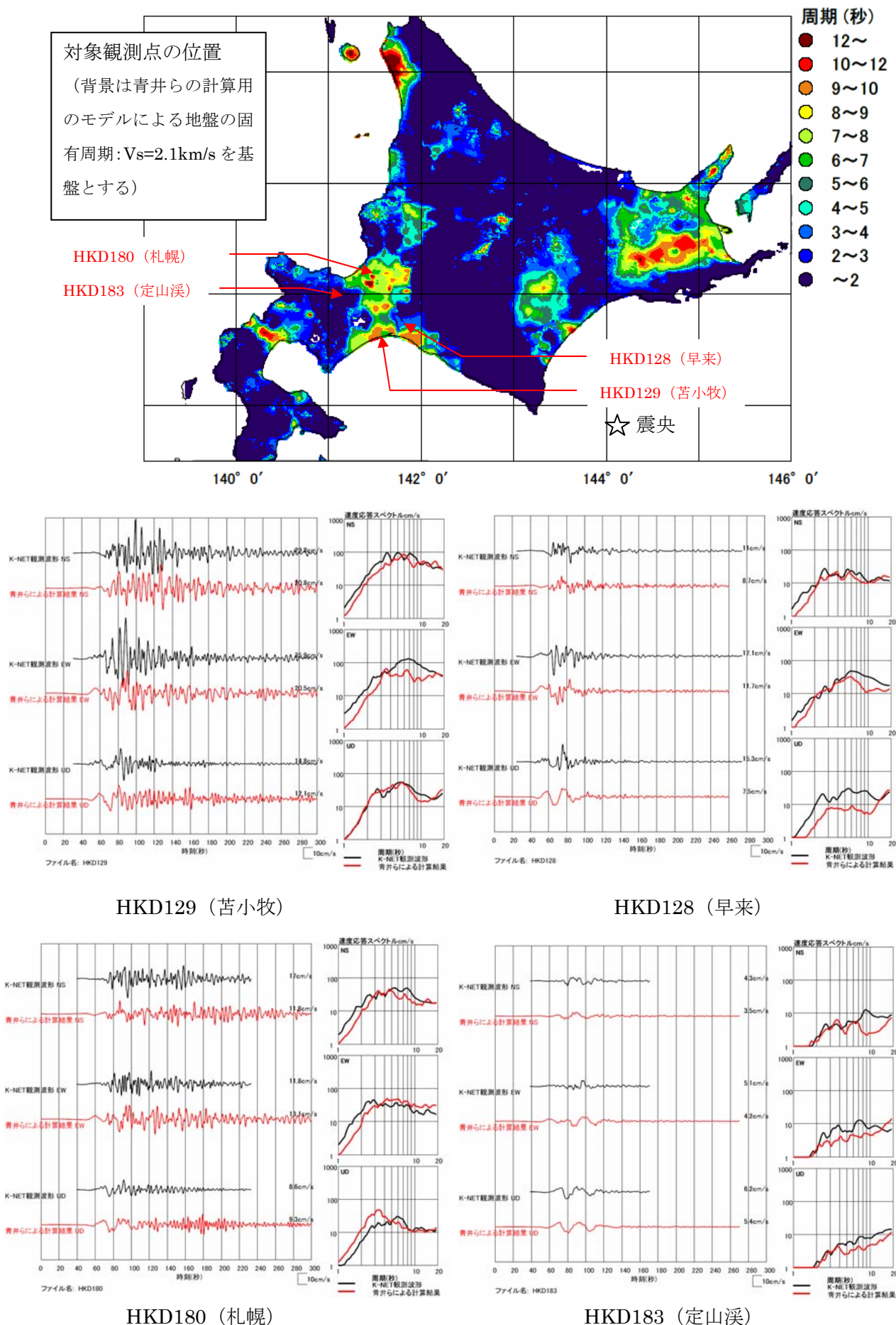
図Ⅱ－14 代表地点における波形と速度応答スペクトル(1)
